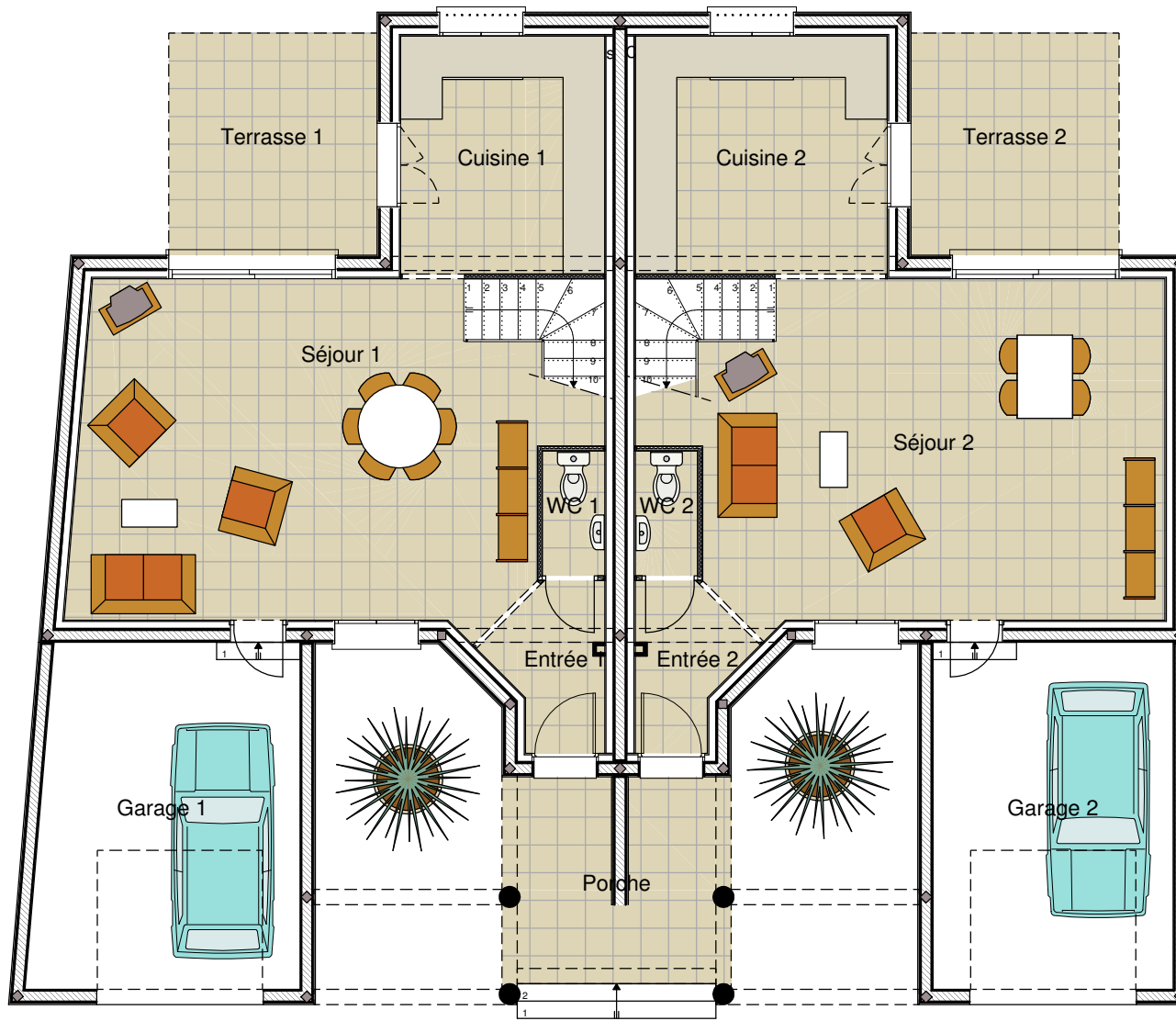
Rez-de-Chaussée
